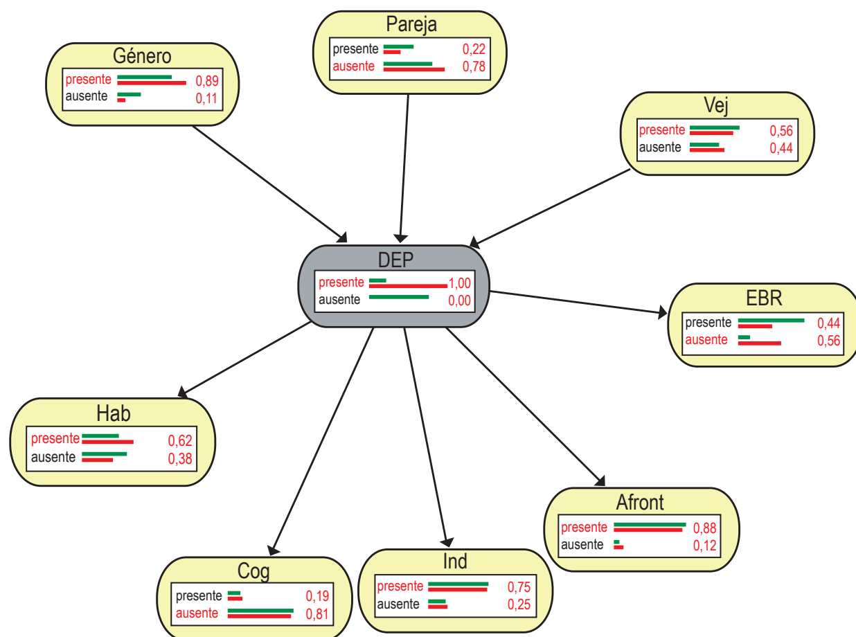
Figura 1. Grafo con SD presente
