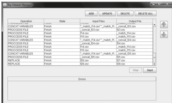
Figura 1. Ventana principal.
